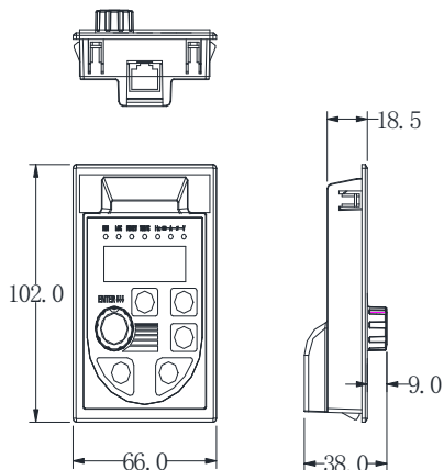
图2-7. 外引键盘带托盘安装尺寸图
