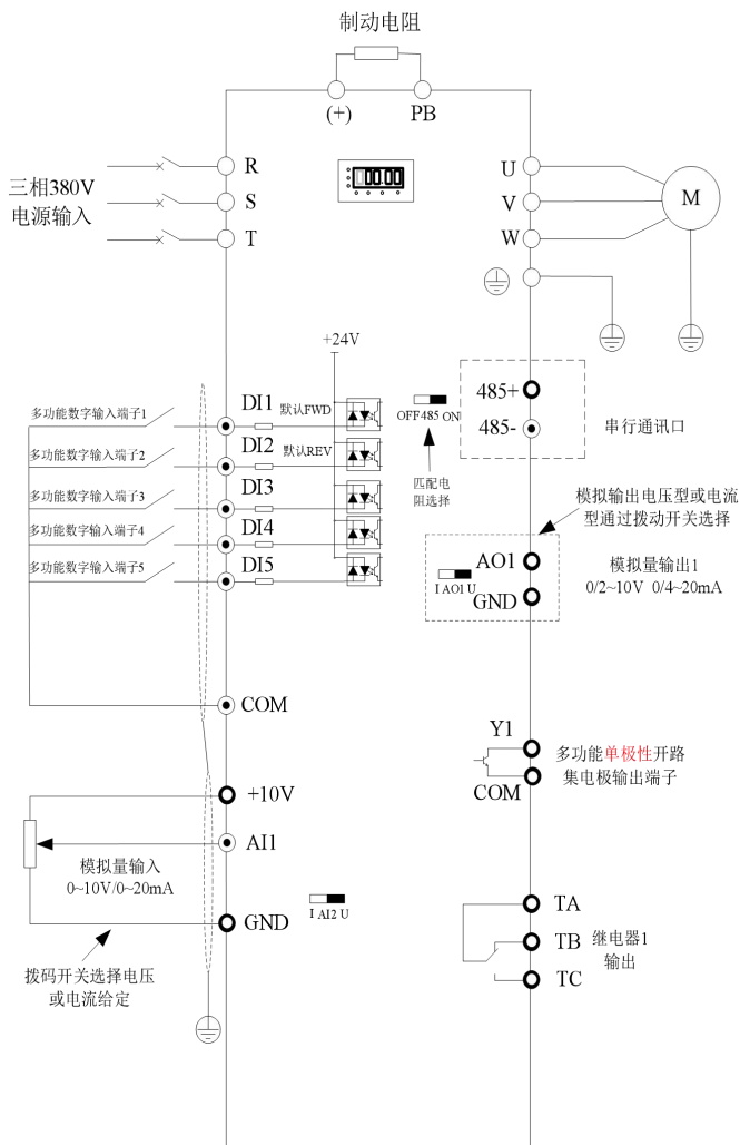
图 3-1. 三相 (380V) 变频器 \leq 9.0\text{kW} (简易型)
