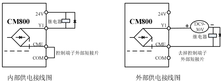
图3-5. 数字输出端子Y1接线示意图
