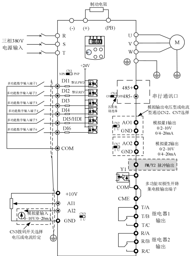
图3-3. 三相变频器 (380V) \cong 11.0kW (通用型)
