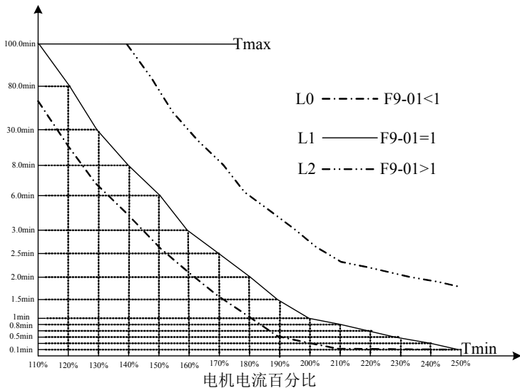
图5-21. 电机过载保护曲线
