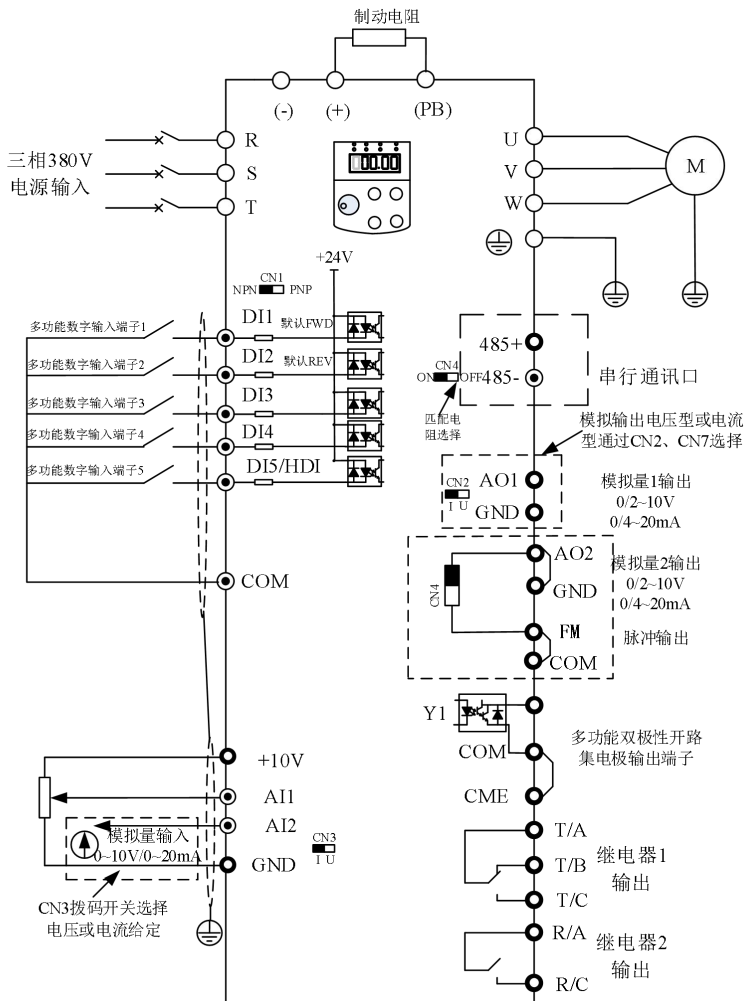
图 3-2. 三相 (380V) 变频器 \leq 9.0\text{kW} (通用型)
