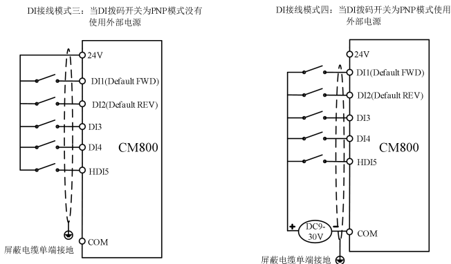
图3-11. 四种不同模式下数字输入端子接线图
