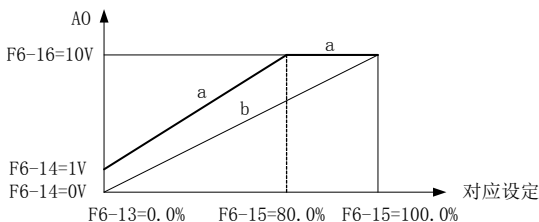
图4-29. AO输出示意图
