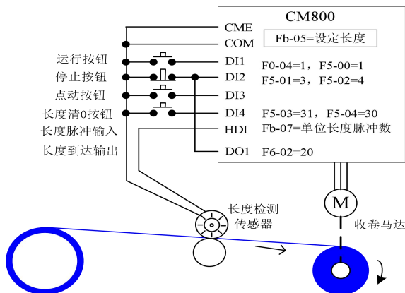
图 4-24. 定长控制功能常见应用举例
