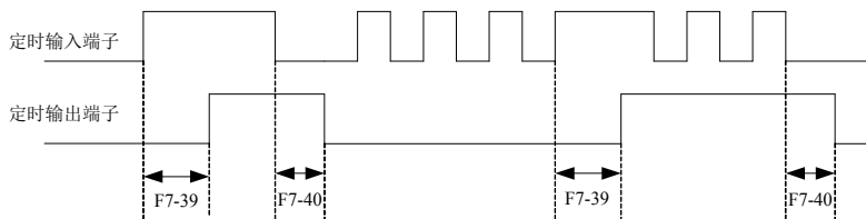
图 5-19. 定时器输入输出动作简图
