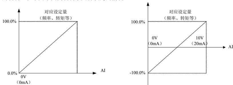
图 5-11. 模拟给定与设定量的对应关系
