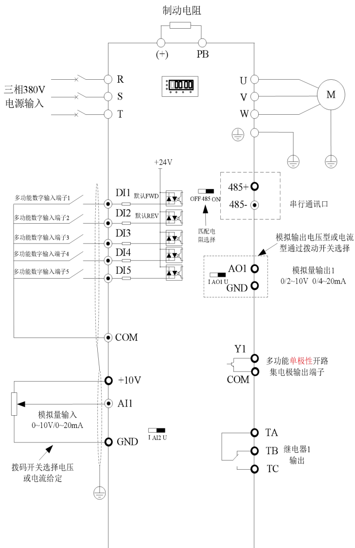
图 3-1. 三相 (380V) 变频器 \leq 9.0\text{kW}
