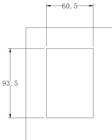
图2-5. 外引键盘带托盘安装开孔尺寸
