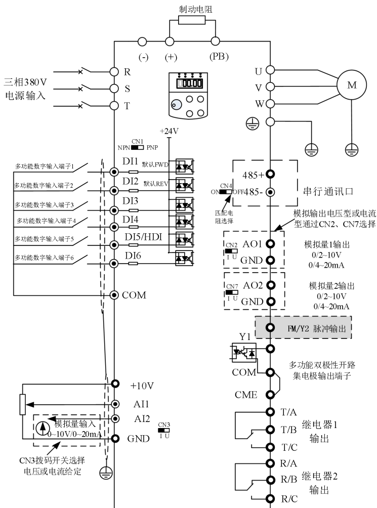
图 3-3. 三相变频器 (380V) \cong 11.0kW
