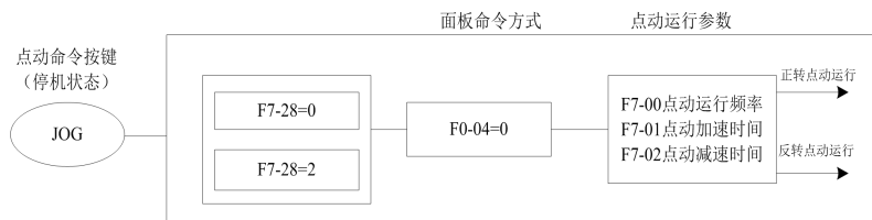
图4-15. 点动参数设定示意图
