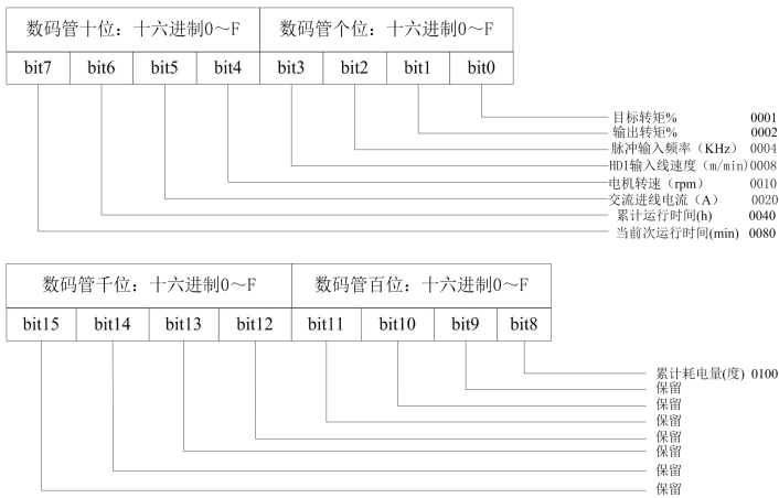
图 6-20. LED 运行显示位对应图
