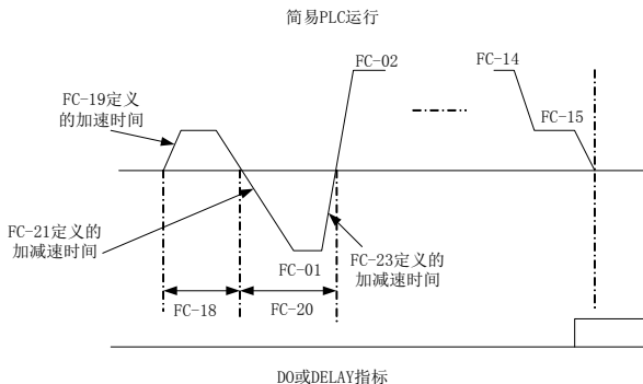
图6-29. 简易PLC示意图
