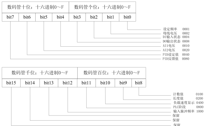
图 6-18. LED 停机显示对应图
