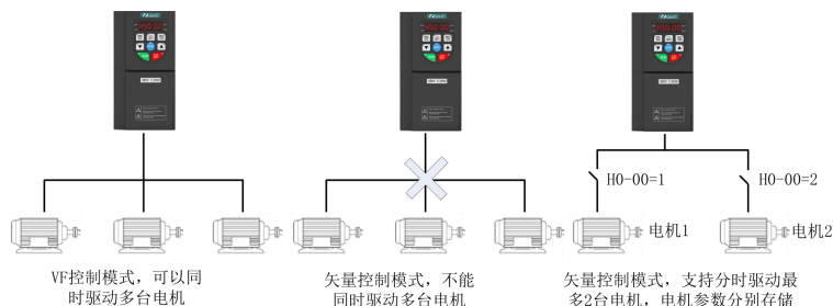
图 4-26. 多组电机的切换
