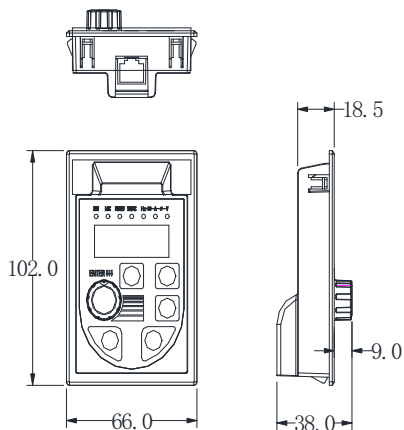
图2-7. 外引键盘带托盘安装尺寸图
