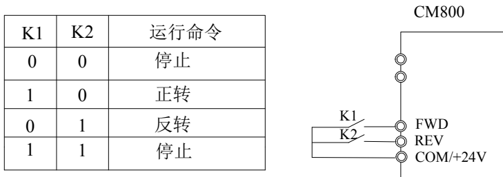
图 6-7. 两线式运转模式 1
