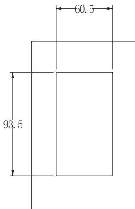
图2-8. 外引键盘带托盘安装开孔尺寸
