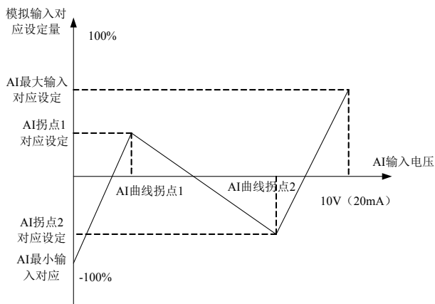
图6-30. 多点曲线对应示意图
