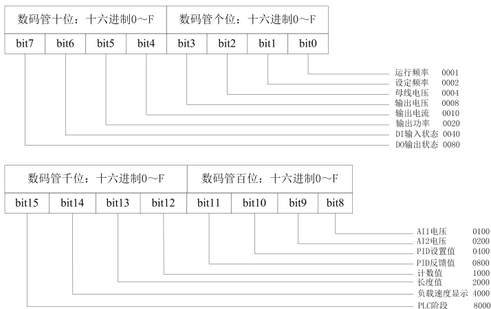
图 6-17. LED 运行显示位对应图
