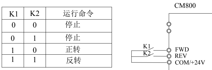
图6-8. 两线式运转模式2
