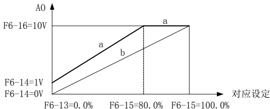
图4-29. AO输出示意图
