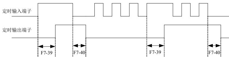
图 6-19. 定时器输入输出动作简图
