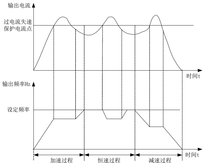
图6-22. 过流失速保护示意图
