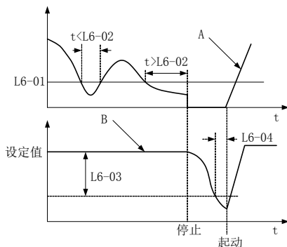
图6-32. 休眠过程频率图
