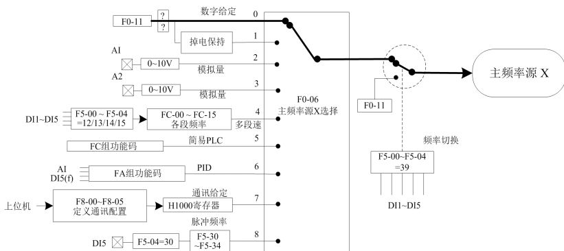
图4-17. 主频率源X设置示意图
