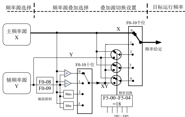
图6-1. 频率源叠加示意图
