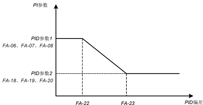
图6-24. PID参数切换
