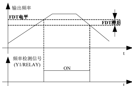
图 6-15. FDT 电平示意图
