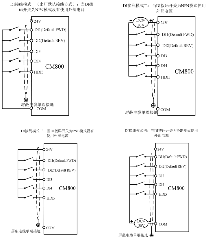
图3-4. 四种不同模式下数字输入端子接线图
