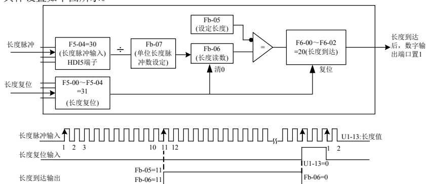
图 4-23. 定长控制模式功能码设置
