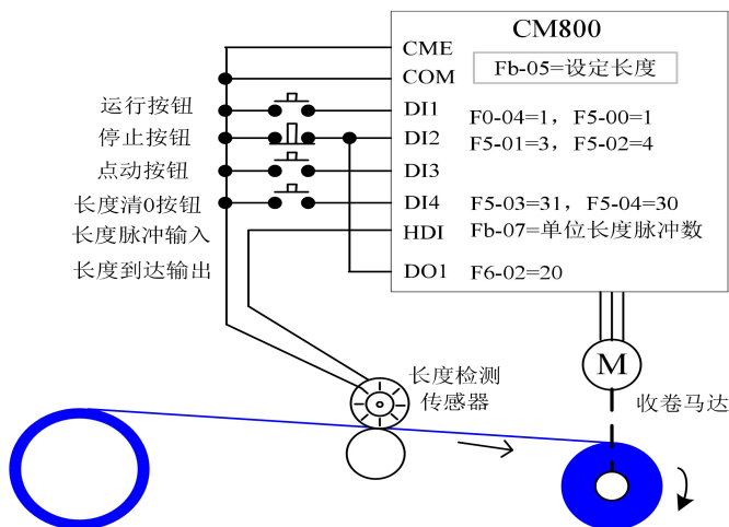
图 4-24. 定长控制功能常见应用举例
