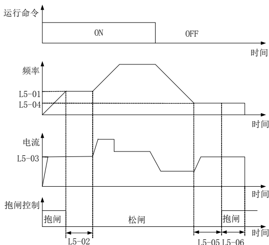
图6-31. 抱闸控制过程图
