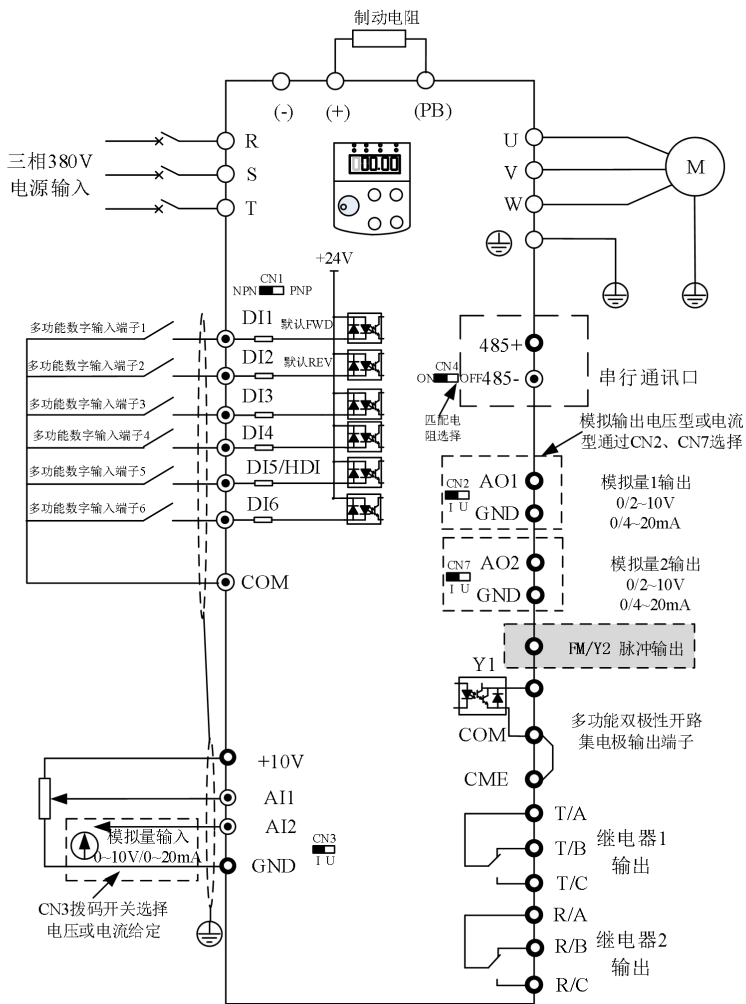
图3-2. 三相变频器 (380V) \geq 11.0\text{kW} (通用型)
