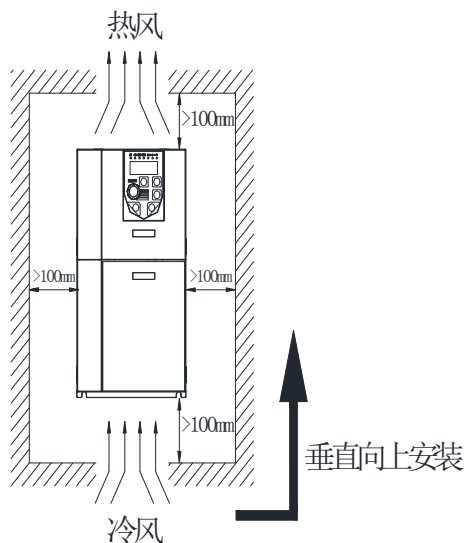
图3-1. 单体安装图
