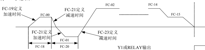
图 6-28. 简易 PLC 示意图
