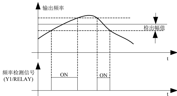
图 6-16. 频率到达检出幅值示意图
