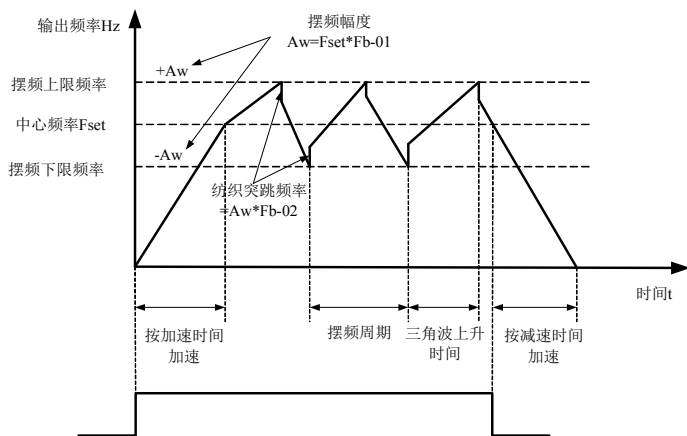
图6-26. 摆频工作示意图
