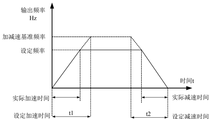
图6-2. 加减速时间示意图
