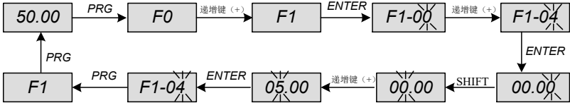
图4-3. 参数设定操作流程图
