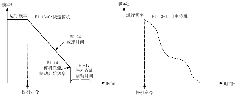
图4-13. 停机示意图
