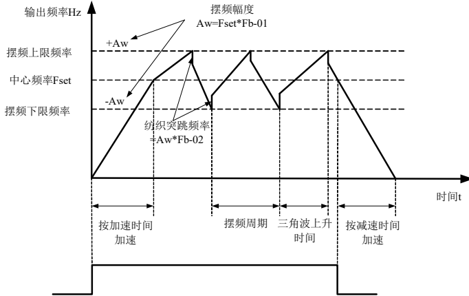
图5-26. 摆频工作示意图
