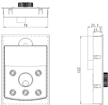
图2-14. 外引键盘带托盘安装尺寸图
