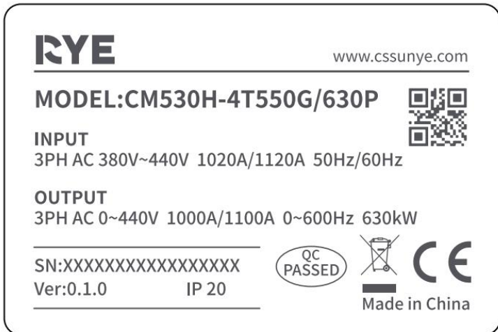
图2-2. 铭牌
