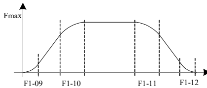
图 5-3. S 曲线加减速示意图
