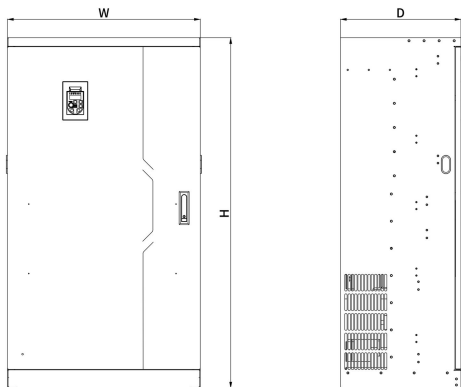
图 2-6. 380V (4T) 355~400kW 变频器外型尺寸及安装尺寸示意图
