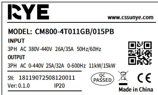
图 2-2. 铭牌
