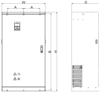
图 2-10. 380V (4T) 160~450kW 变频器外型尺寸及安装尺寸示意图
