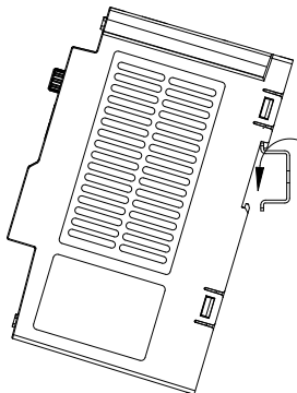
图 5-11 导轨安装示意图 2
