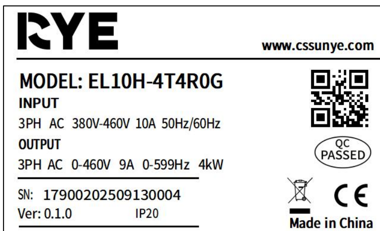
图 1-2 三相 4kW 铭牌示例
