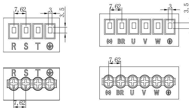
输入端子
