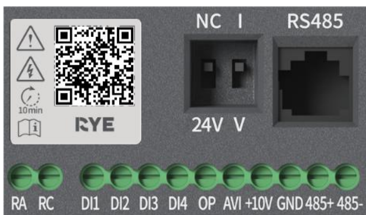
图 6-3 控制回路端子布置图【EL10H】
