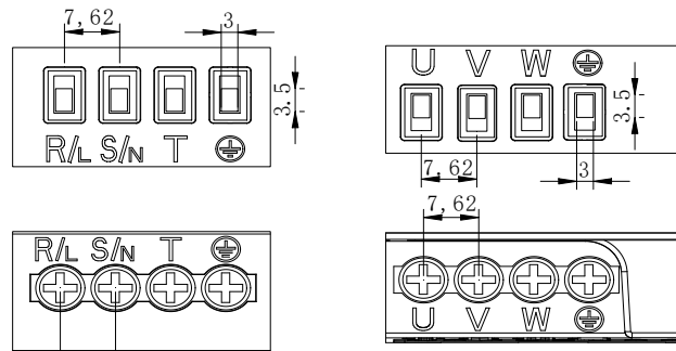
输入端子
