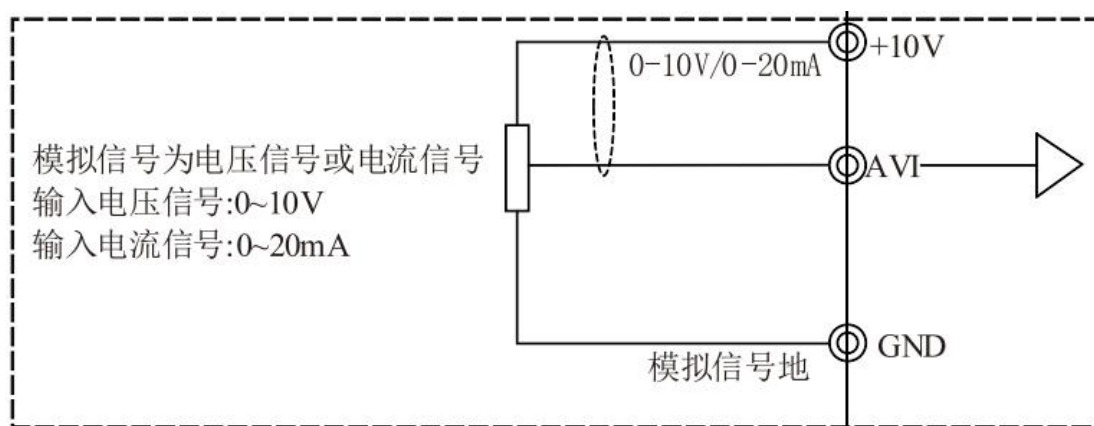
图 6-4 模拟量输入端子接线示意图
