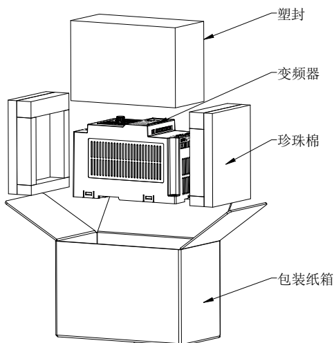
图 5-8 包装清单
