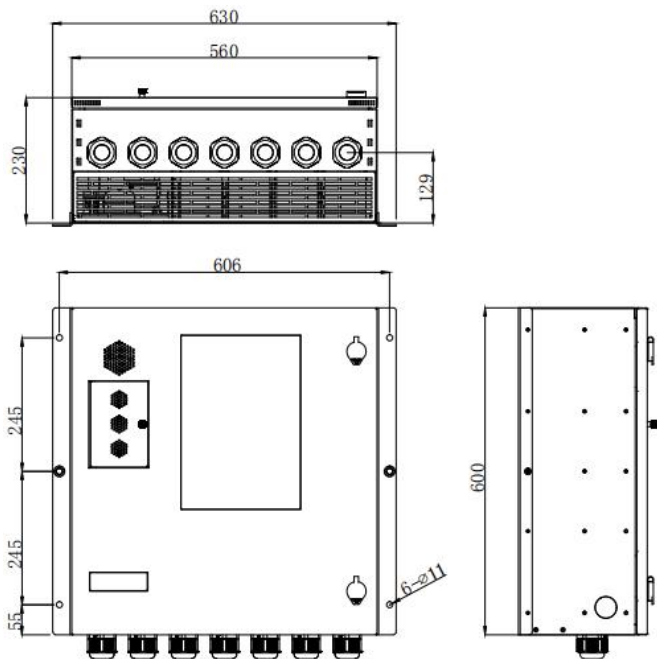
BM300B-055 / 075 尺寸
