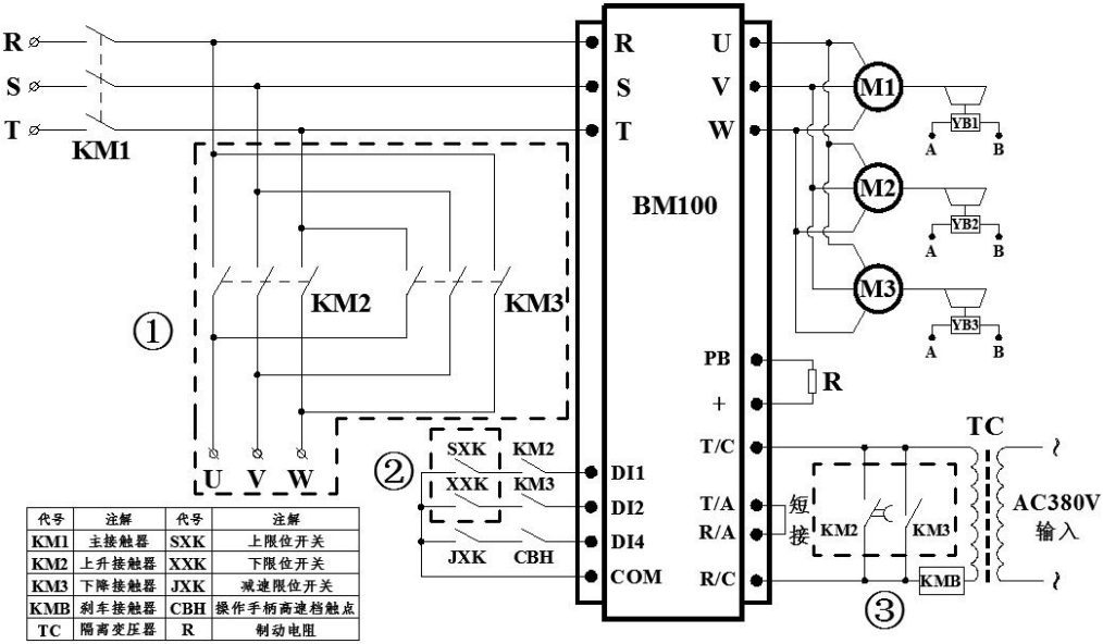
BM100-037 变频改造接线示意图
