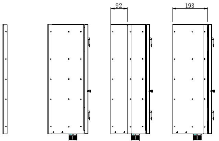
安装固定条
