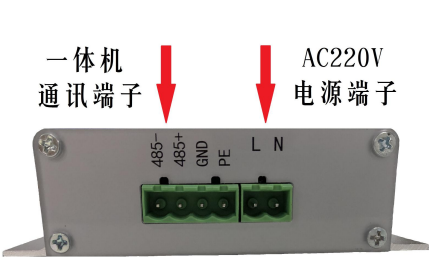
接线端子
