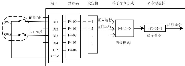
图4-4. 端子控制启停示意图
