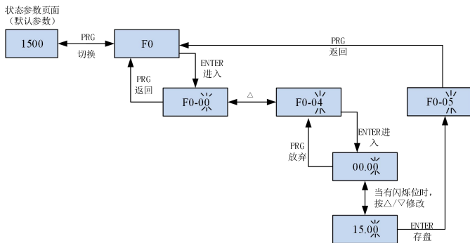
图4-3. 参数设定操作流程图
