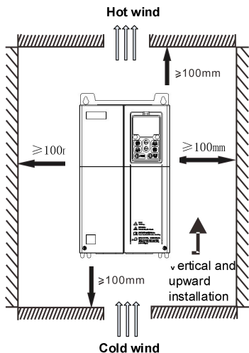
图3-1. 单体安装图
