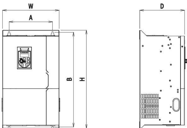
图 2-4. 30~45kW 钣金机箱尺寸及安装尺寸示意图
