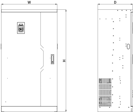
图 2-6. 380V (4T) 355~400kW 变频器外型尺寸及安装尺寸示意图
