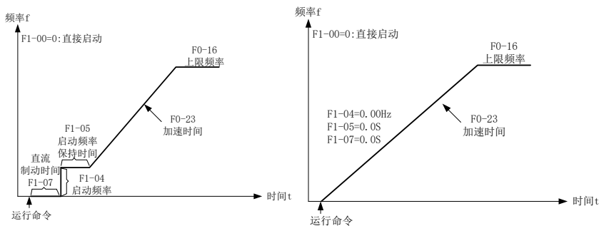
图6-7. 直接启动示意图
