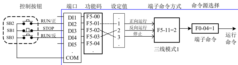
图6-5. 端子控制启停示意图
