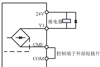
内部供电接线图
