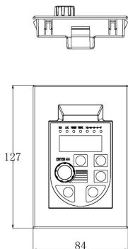
图2-7. 外引键盘带托盘安装尺寸图
