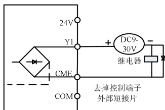
外部供电接线图
