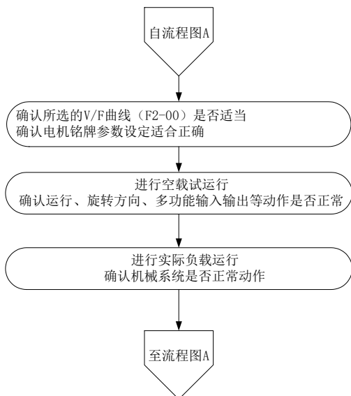
图 6-3. V/F 控制方式运行步骤
