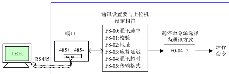
图6-6. 通讯控制启停示意图
