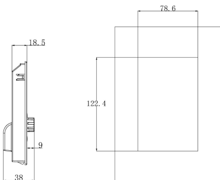
图2-8. 外引键盘带托盘安装开孔尺寸
