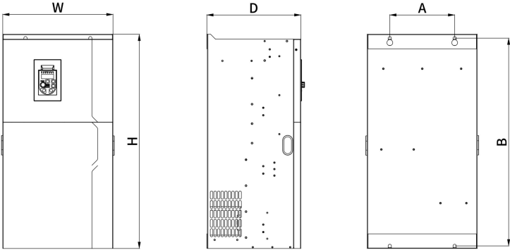
图 2-5. 380V (4T) 55~315kW 变频器外型尺寸及安装尺寸示意图
