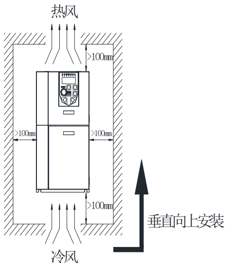
图3-1. 单体安装图
