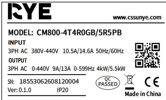
图 2-2. 铭牌
