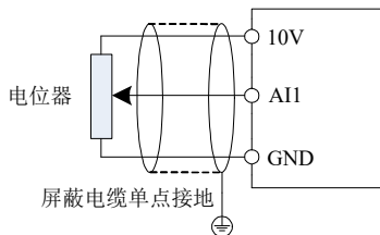
图 3-3. 模拟量输入端子接线示意图
