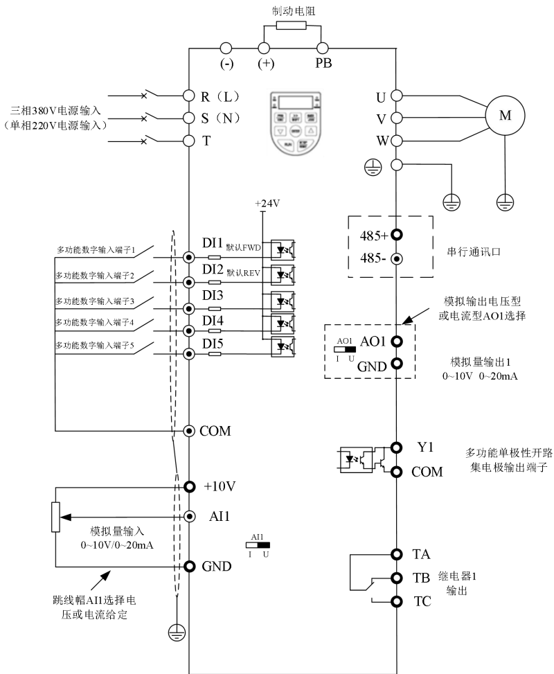
图 3-1. 三相 (380V) 变频器 \leq 9.0\text{kW}
