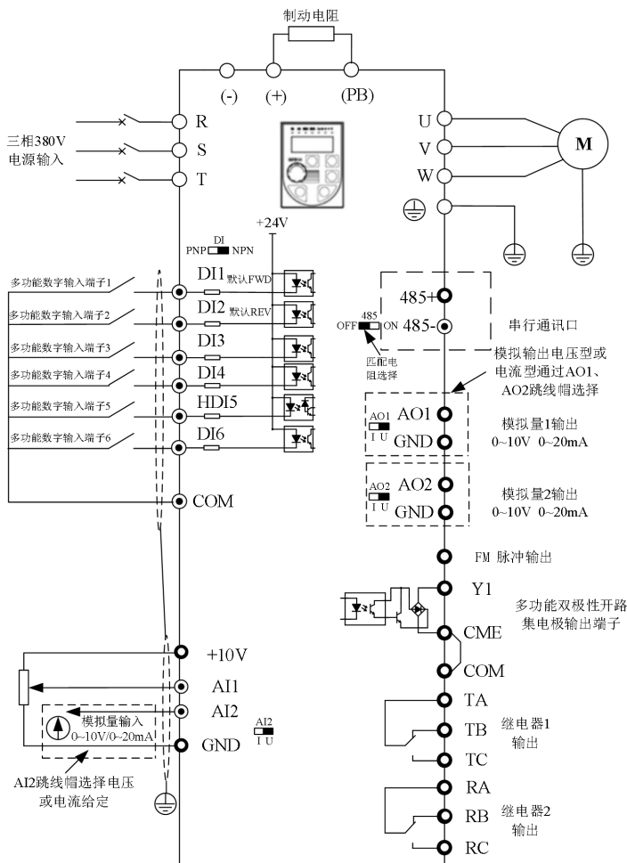
图3-2. 三相变频器（380V）11kW及以上
