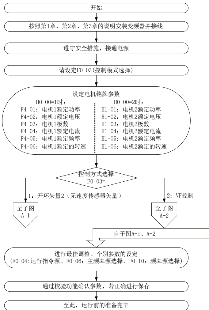
图 6-1. 运行前的基本步骤
