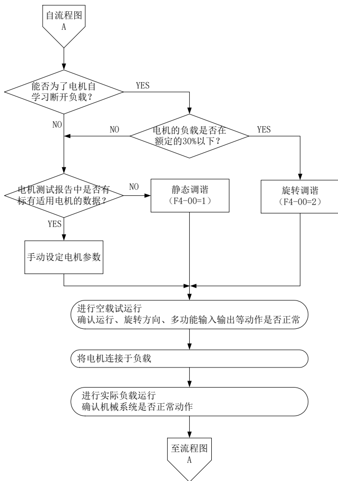
图 6-2. 开环矢量控制方式运行步骤
