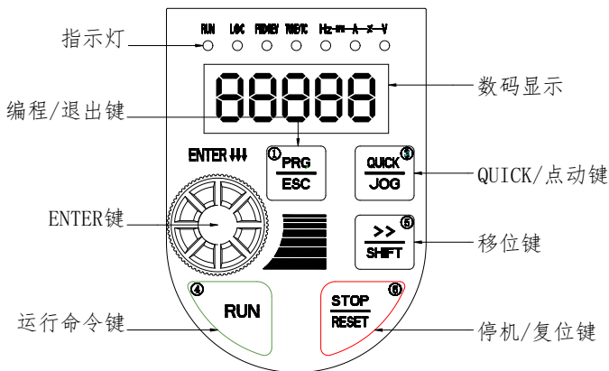
图4-1. LED旋钮键键盘（11.0kW及以上变频器标准配置）（含11KW）
