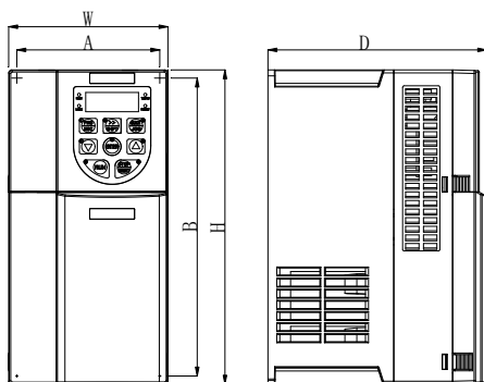
图2-3. 22kW及以下塑胶外形尺寸及安装尺寸示意图
