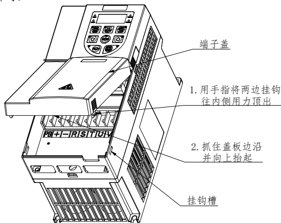
图3-5. 塑胶外壳端子盖拆卸图
