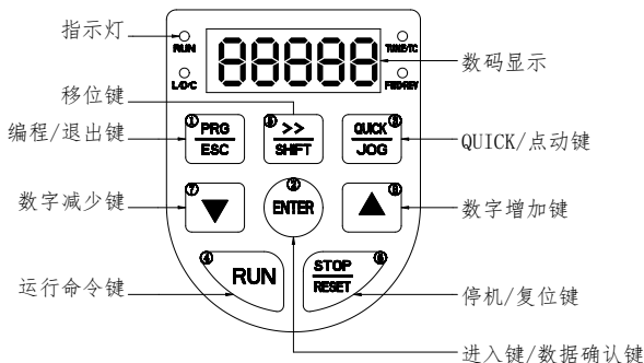
LED纯按键键盘（9.0kW及以下变频器标准配置）
