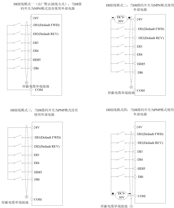
图3-4. 四种不同模式下数字输入端子接线图
