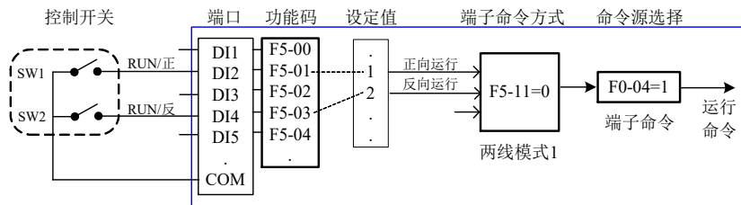
图6-4. 端子控制启停示意图
