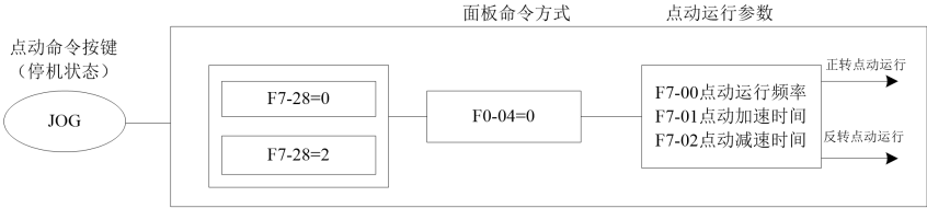
图4-15. 点动参数设定示意图
