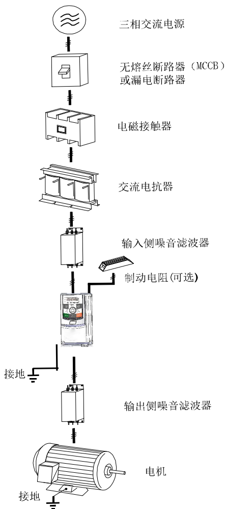
图 1 与外围机器的连接示例
