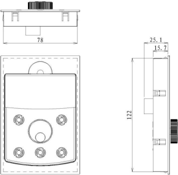
图2-14. 外引键盘带托盘安装尺寸图
