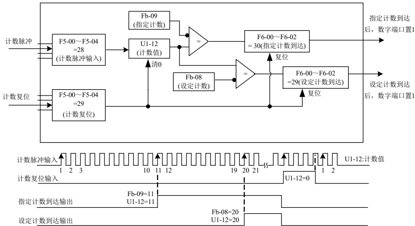
图 4-25. 计数模式功能码设置
