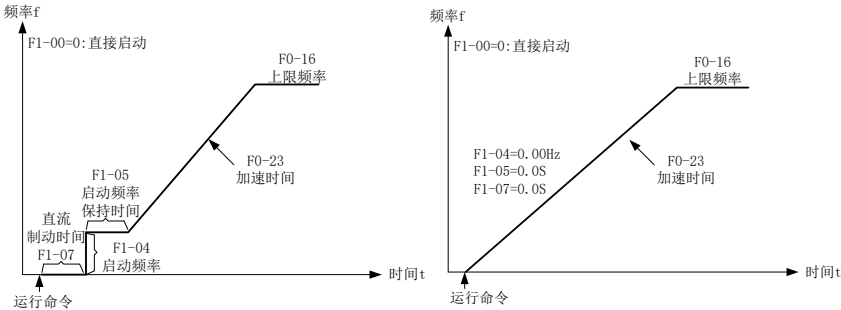
图4-11. 直接启动示意图
