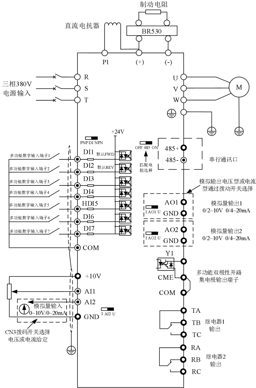
图 3-9. (4T/7T) 75kW 及以上三相变频器
