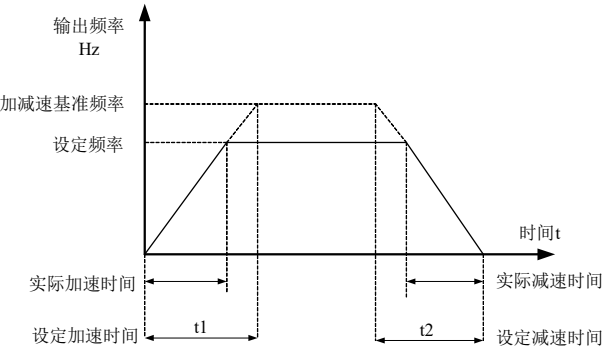
图5-2. 加减速时间示意图
