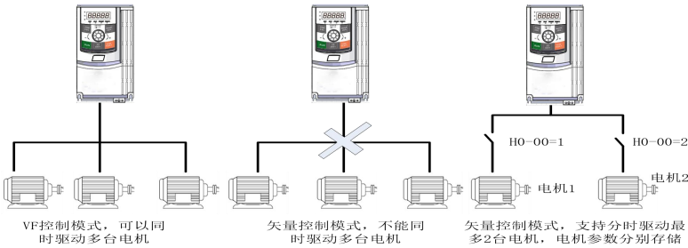
图 4-26. 多组电机的切换
