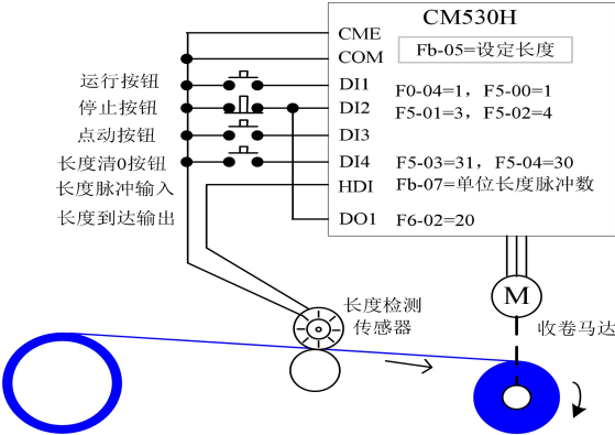
图 4-24. 定长控制功能常见应用举例
