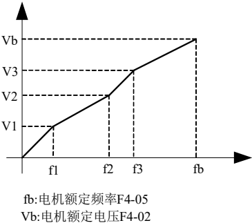
图 5-5. V/F 曲线设定示意图
