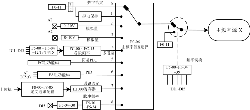
图4-17. 主频率源X设置示意图
