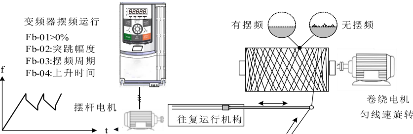
图4-20. 摆平运用设置示意图
