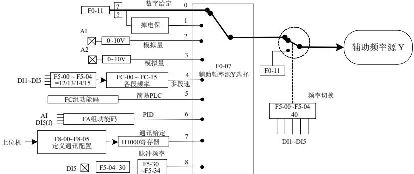
图4-18. 辅助频率源Y设置示意图
