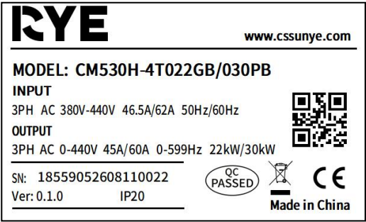
图2-2. 铭牌
