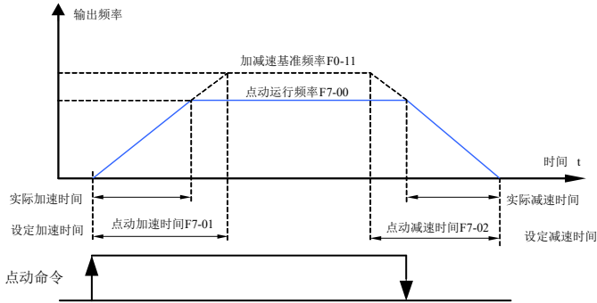
图4-14. 点动运行示意图
