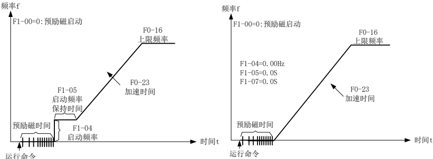
图4-12. 预励磁启动示意图
