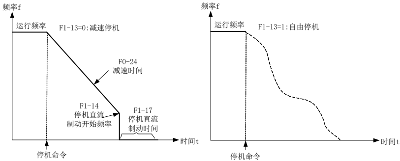
图4-13. 停机示意图
