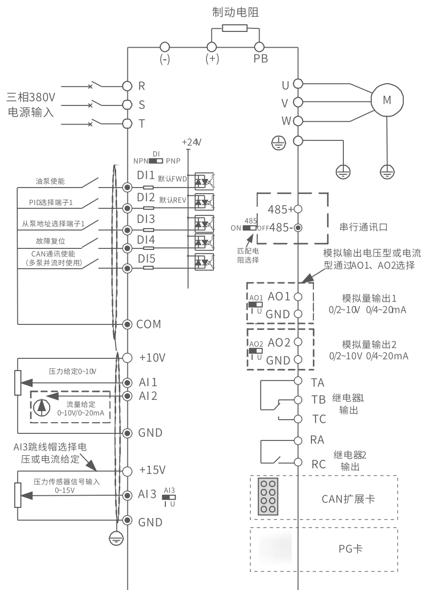
接线方式图
