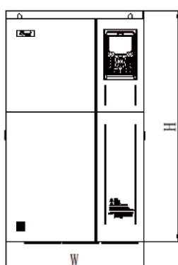
11~22kW塑壳机箱外形尺寸及安装尺寸示意图
