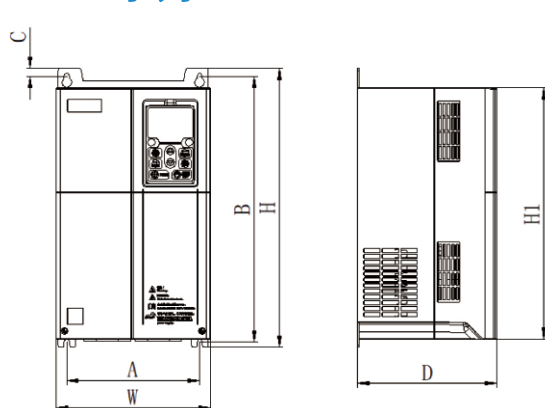
11~22kW塑壳机箱外形尺寸及安装尺寸示意图
