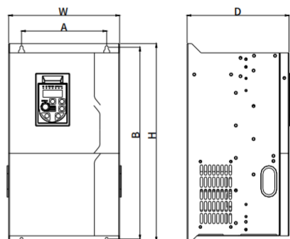
图4. 30kW以上钣金机箱尺寸及安装尺寸示意图
