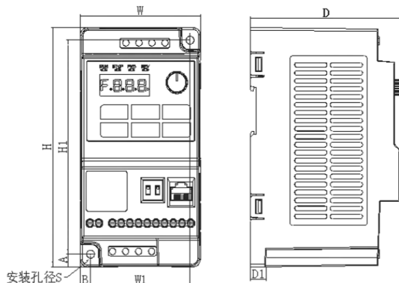
外形及安装尺寸示意图
