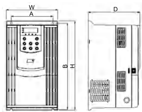
11 ~ 18KW塑壳机箱外形尺寸及安装尺寸示意图
