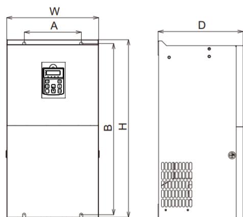
45 ~ 132KW变频器外型尺寸及安装尺寸示意图
