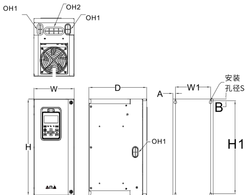
(C5) 380V(4T) 37~45kW钣金机箱外形尺寸及安装尺寸示意图
