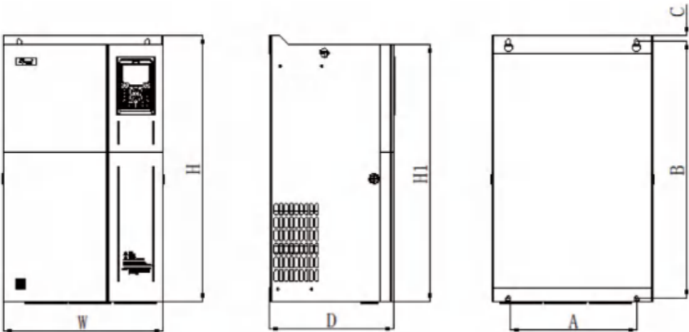
45 ~ 132kW变频器外型尺寸及安装尺寸示意图
