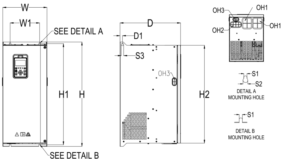
图2-4 (C6~C8) 380V(4T) 55~185kW变频器外型尺寸及安装尺寸示意图
