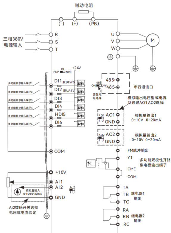
图2.三相变频器（380V）11kW及以上
