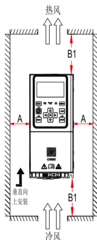
C2~C8机型壁挂安装示意图
