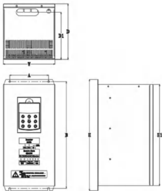
200kW及以上制动单元
