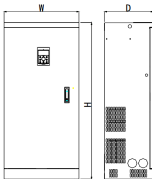
380V(4T) 160 ~ 500kW变频器 外型尺寸及安装尺寸示意图
