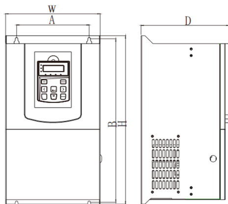
22 ~ 37KW机箱外形尺寸及安装尺寸示意图
