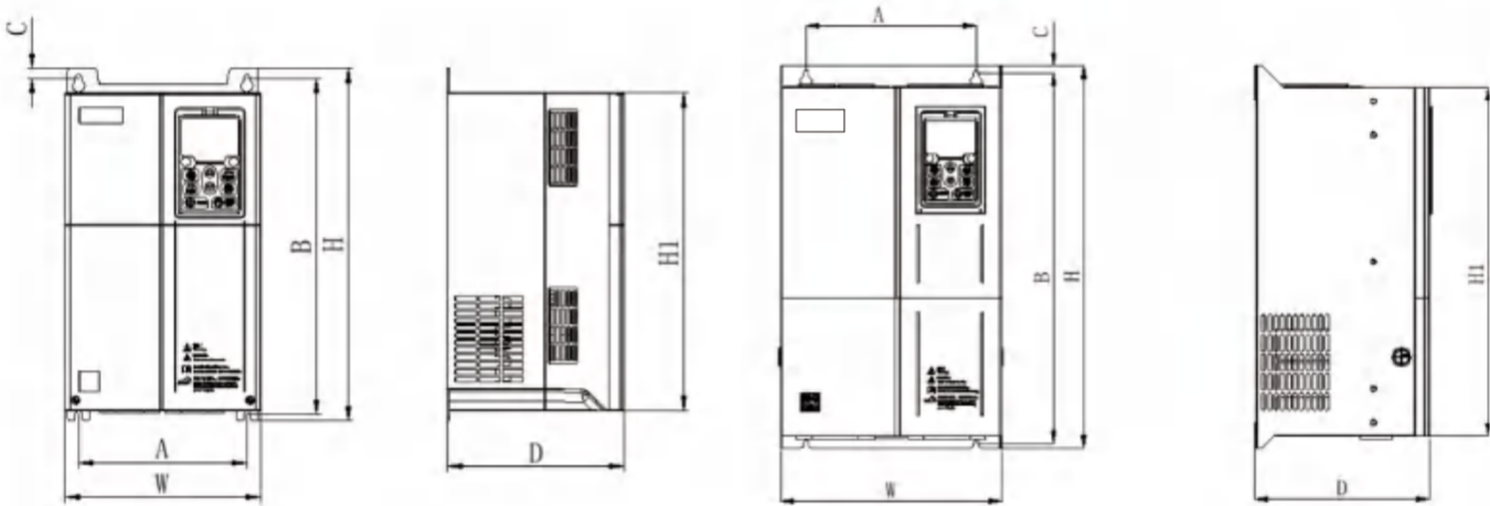
11 ~ 22kW塑壳机箱外形尺寸及安装尺寸示意图
