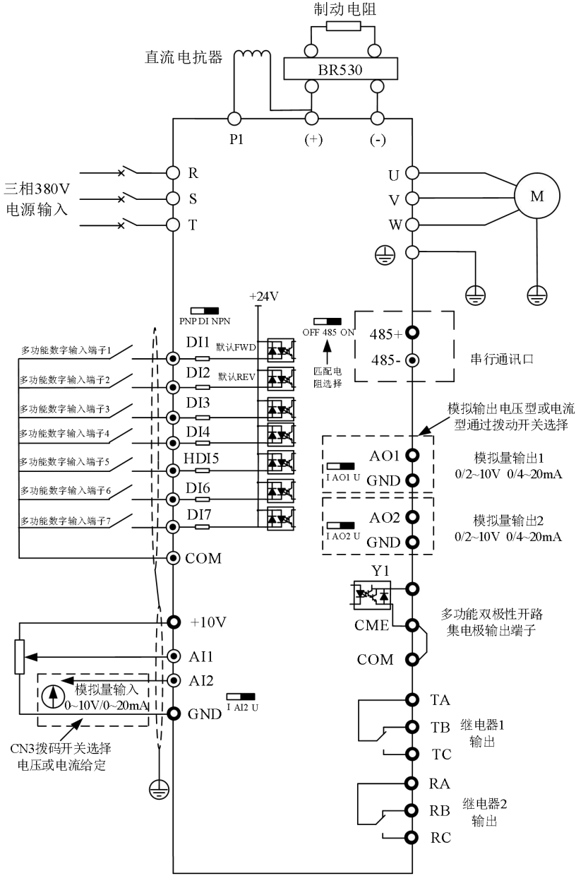
图 3-8. (4T/7T) 75kW 及以上三相变频器
