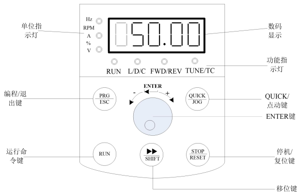
图4-1. 操作面板示意图(标配LED纯按键键盘)
