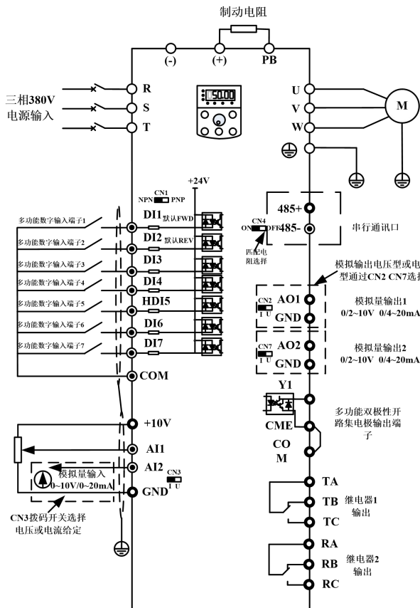
图 3-1. 30kW 以下三相变频器
