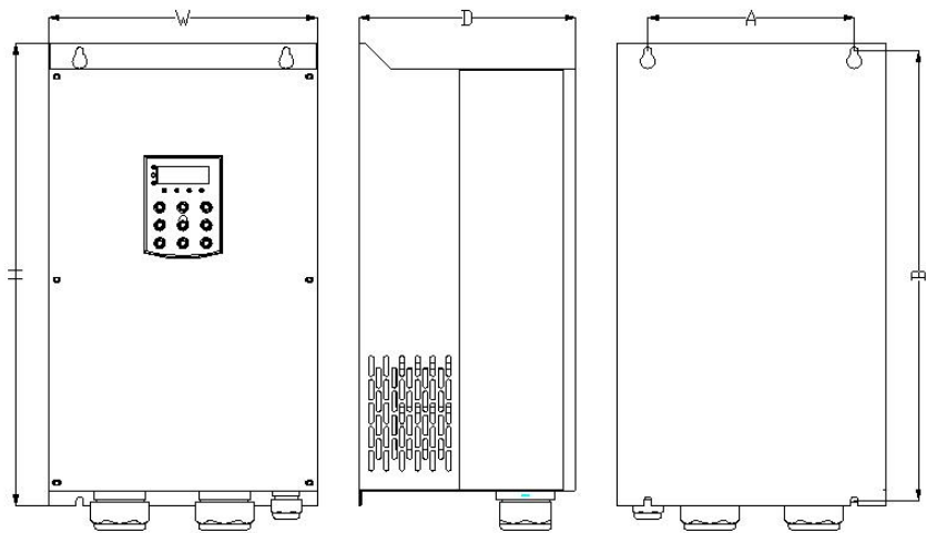
图 2-4. 380V (4T) 9kW~37kW 外形尺寸及安装尺寸示意图
