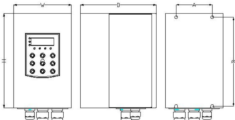
图 2-3. 380V (4T) 1.5kW~7.5kW 外形尺寸及安装尺寸示意图
