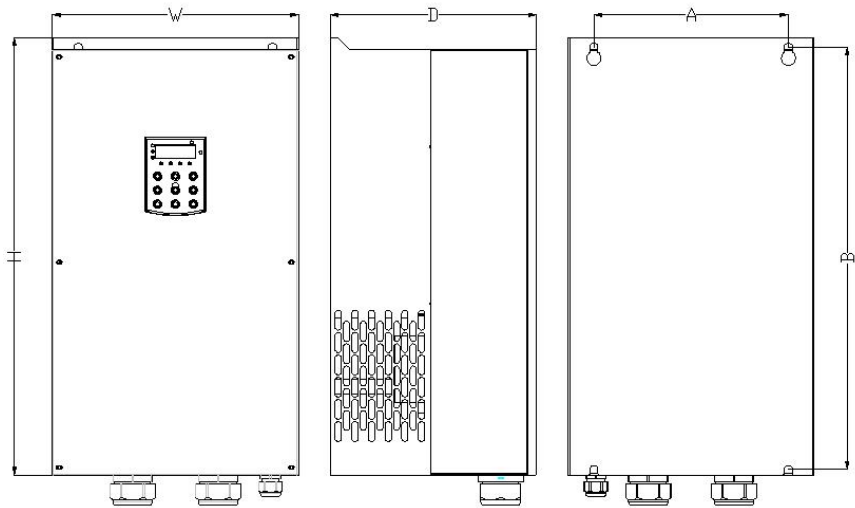
图 2-4. 380V (4T) 9kW~37kW 外形尺寸及安装尺寸示意图
