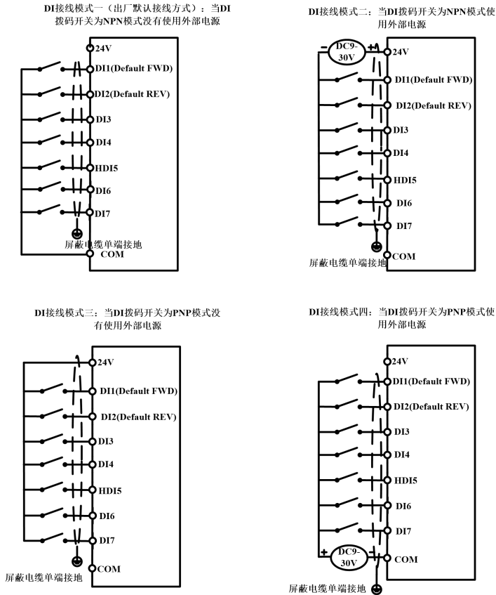
图3-4. MH600变频器四种不同模式下数字输入端子接线图
