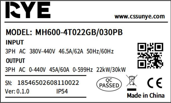
图2-2. 铭牌
