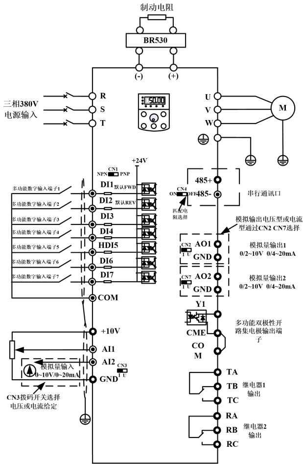
图 3-2. 37kW 以上三相变频器
