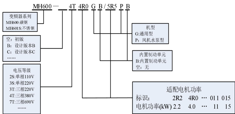
图2-1. 命名规格
