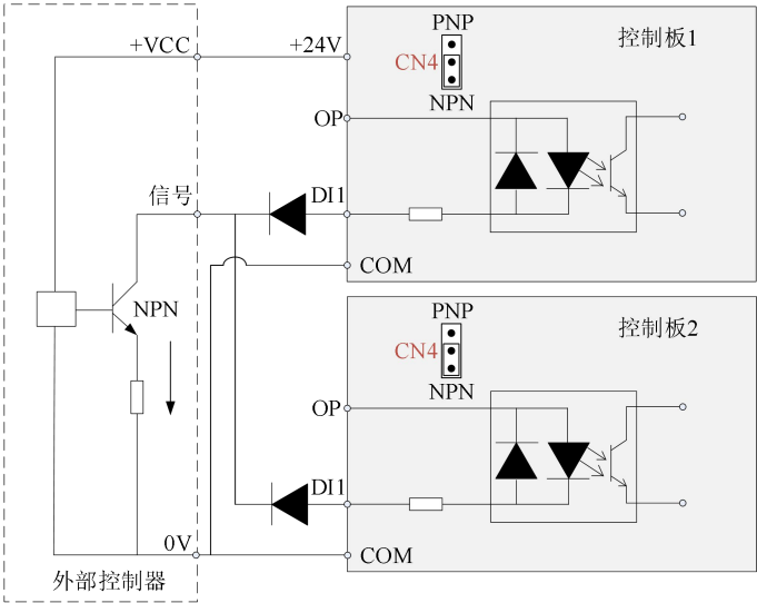
图3-8. 多台伺服驱动器DI端子并接漏型接线方式
