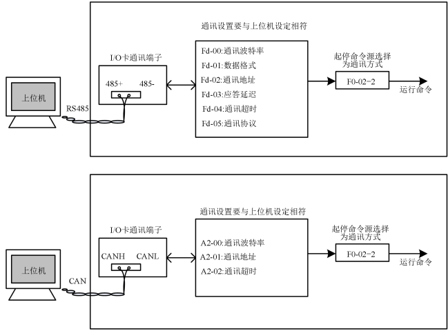
图4-5. 通讯控制启停示意图
