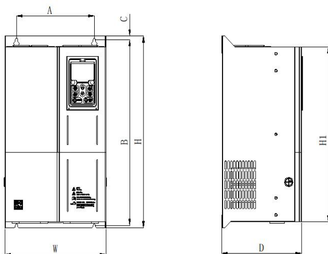
图 2-5. 30-37kW 钣金机箱外形尺寸及安装尺寸示意图
