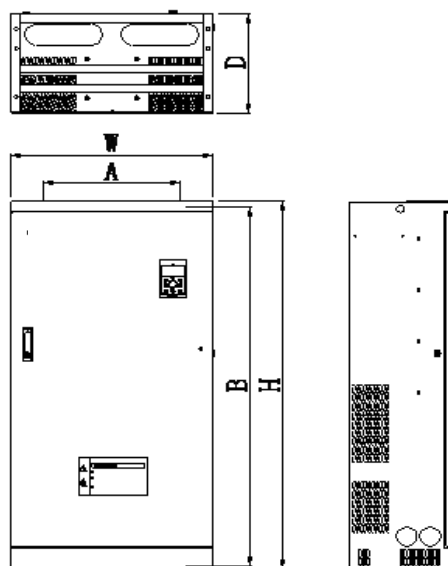
图 2-7. 160~400kW 变频器外型尺寸及安装尺寸示意图
