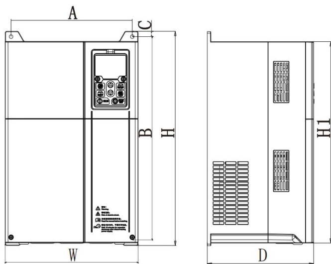
图 2-3. 11~22kW 塑壳机箱外形尺寸及安装尺寸示意图
