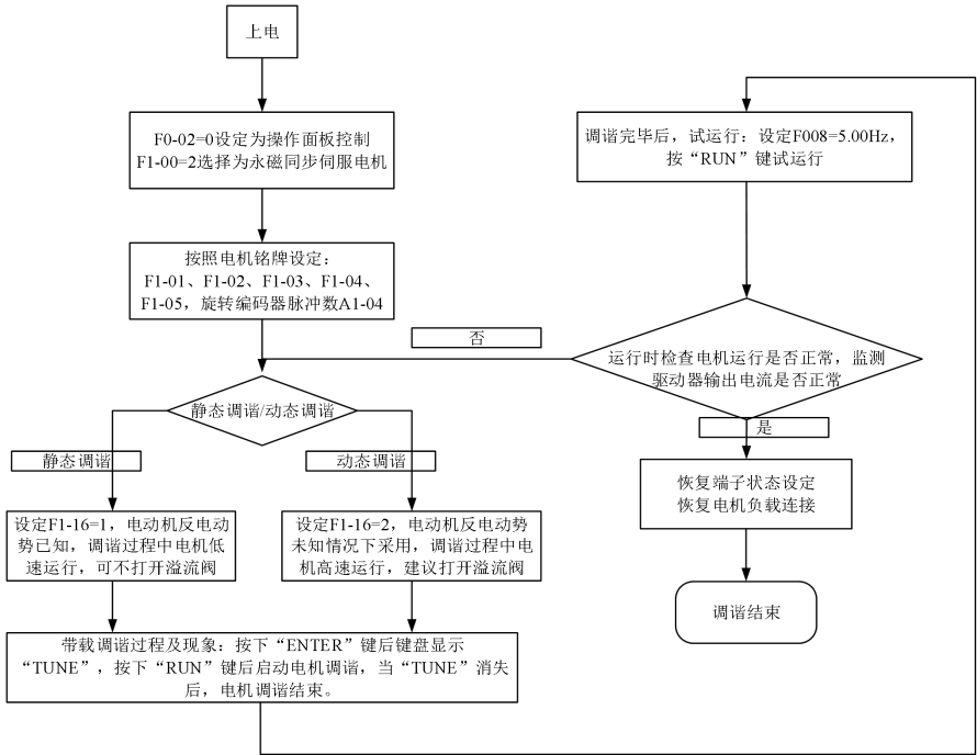
图 5-2 电机参数自学习示意图
