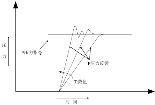
图 5-4 油压 PID 积分时间
