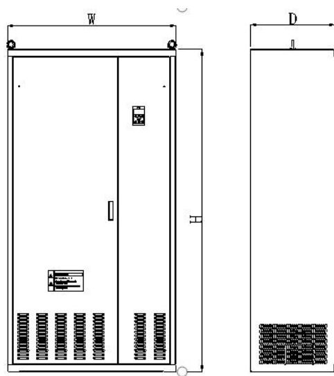
图 2-8. 450~500kW 变频器外型尺寸及安装尺寸示意图
