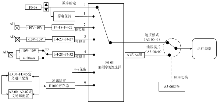
图4-6. 频率给定方式
