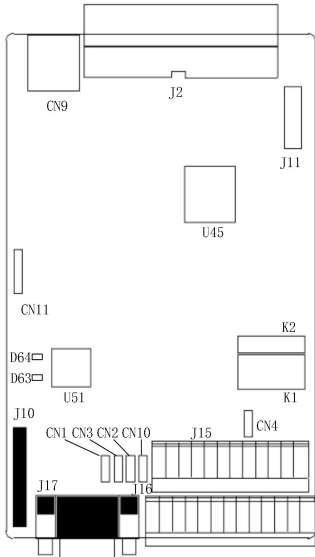
图3-5. 主控板正视图的接线端子及接插件布局图
